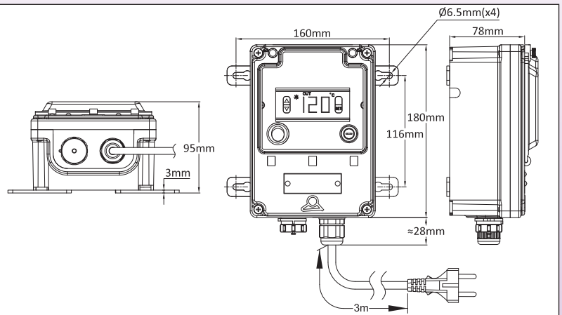
Modelo con conector impermeable de 5 vías
