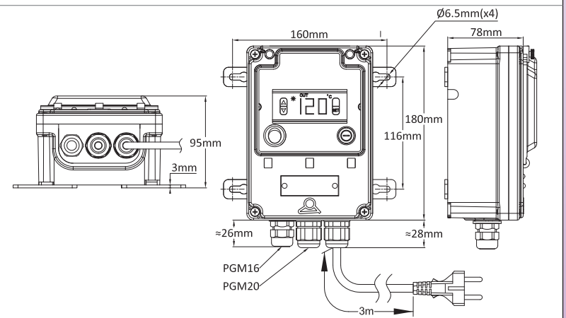
Modelo con 3 glándulas de cable
